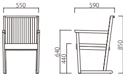
脚置きステンレス HL仕上
